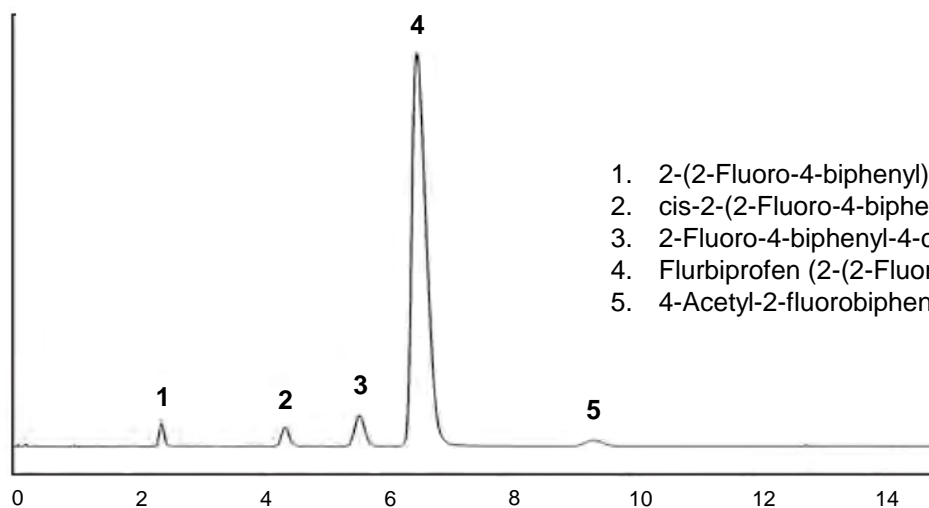
Flurbiprofen
